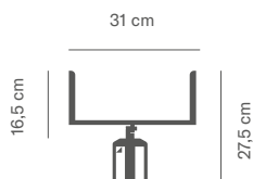
Porta Cartel BASIC A4 H
