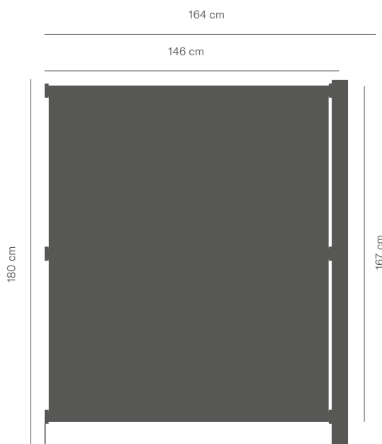
PLAFÓN DOBLE (Extensión)
