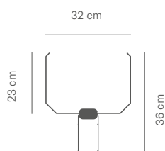
Porta Cartel TERMINAL A4 H
